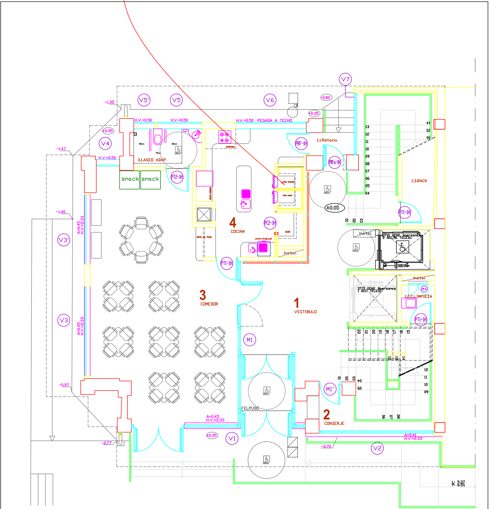
PLANTA BAJA (CENTRO DE DÍA)
