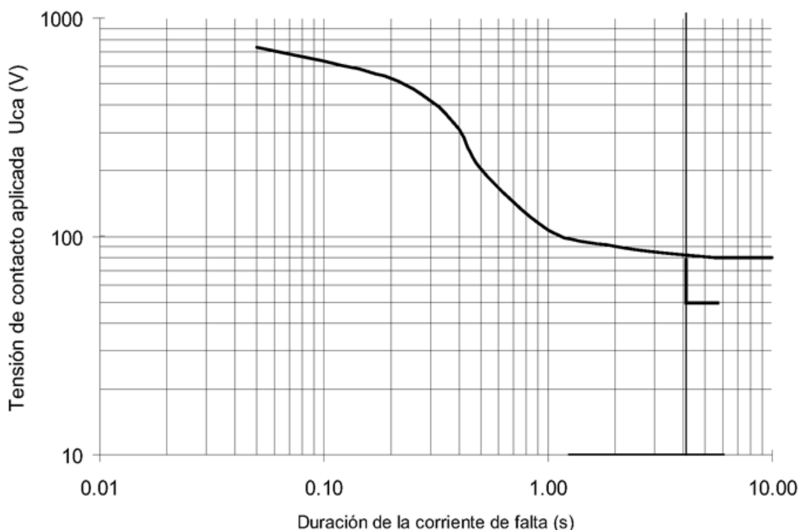
Figura 1. Valores admisibles de la tensión de contacto aplicada U_{ca} en función de la duración de la corriente de falta
